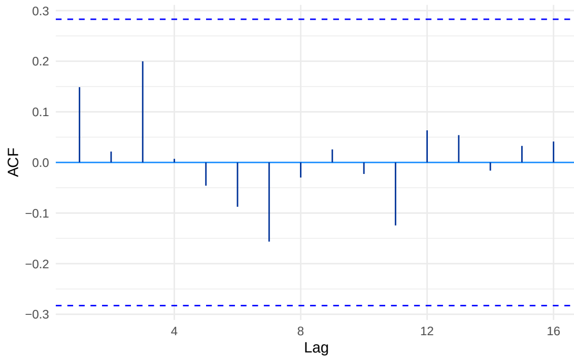
Autocorrélation des résidus (ACF)
