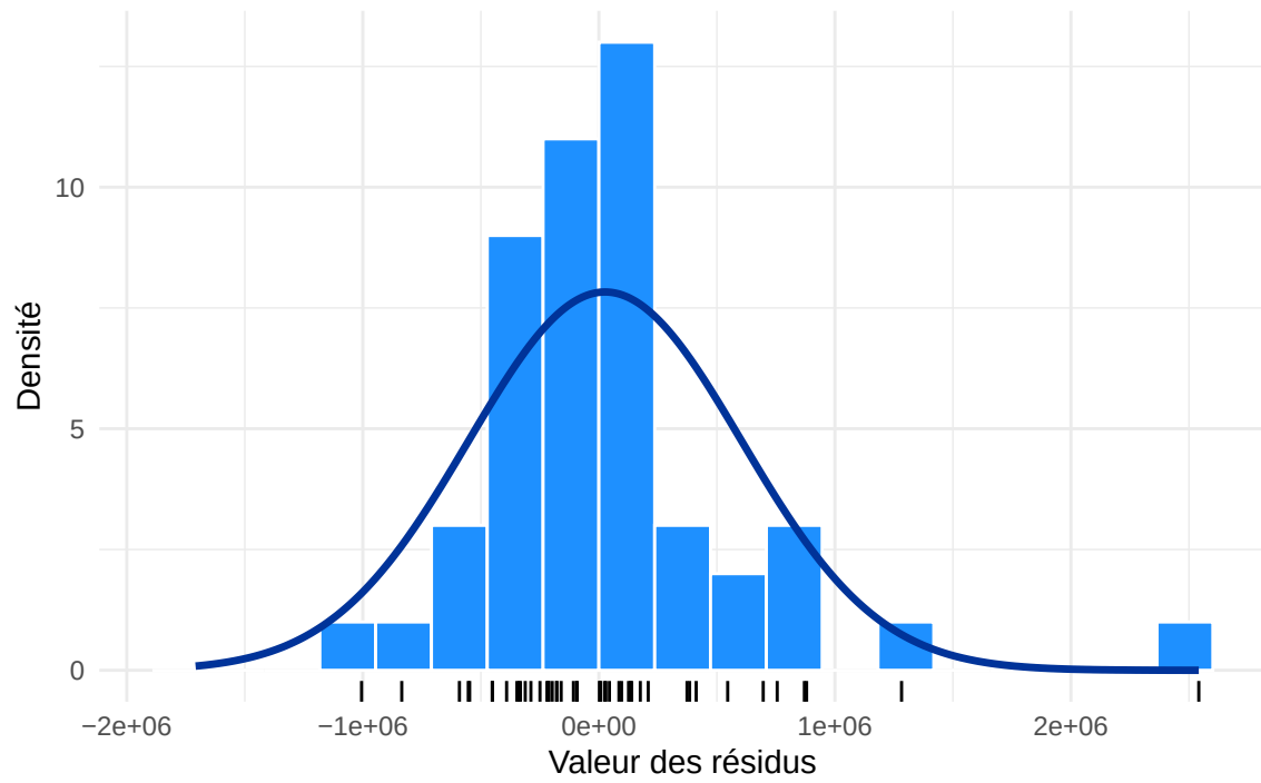
Distribution des résidus
